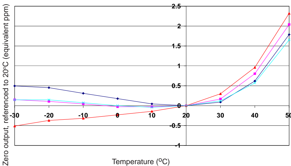
图4 零点温度特性
